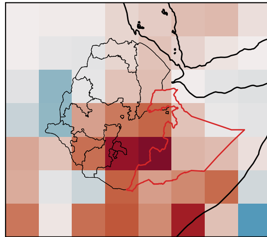
2021 MAM rainfall anomaly
