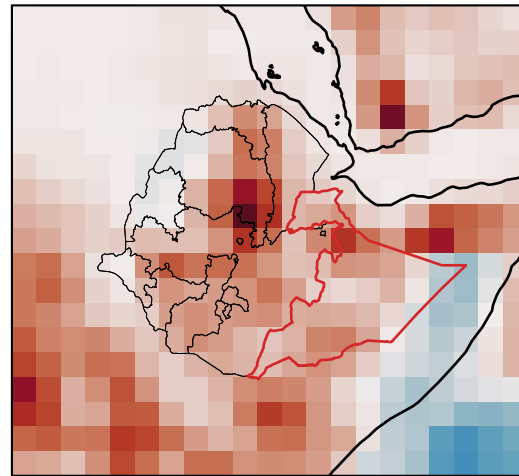
2000 MAM rainfall anomaly
