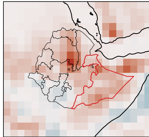
2007 MAM rainfall anomaly
