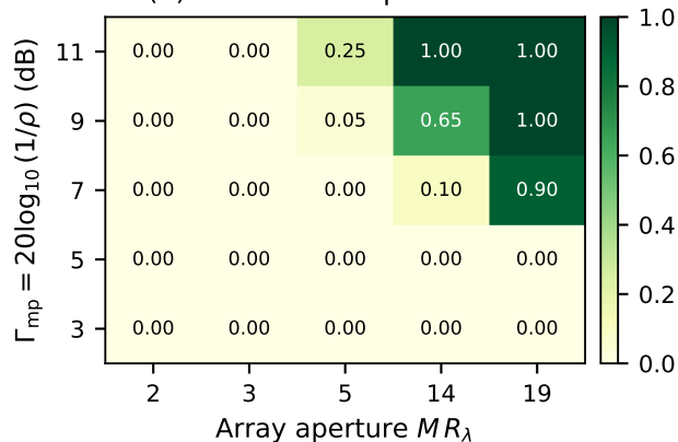
(d) Intermittent transmission
