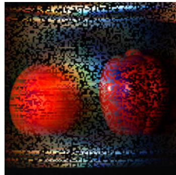
box-legal u (POCS) res 2e-06
