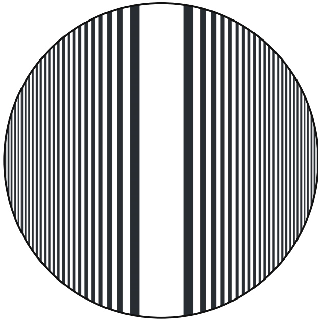
(b) 线型波带片
