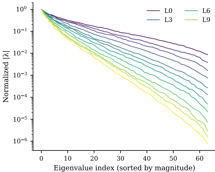
GL + (K): Eigenvalue Spectra
