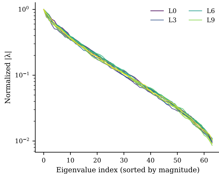
Mixed \pm : Eigenvalue Spectra
