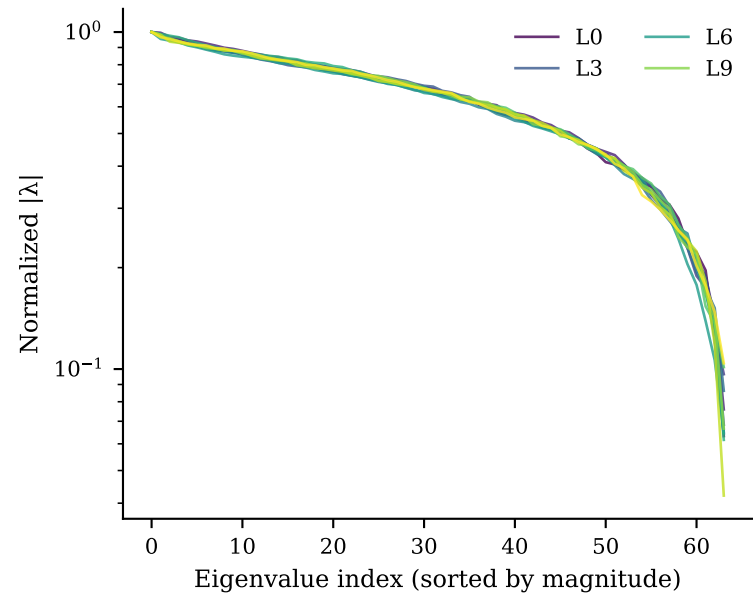
Random: Eigenvalue Spectra
