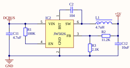
DC-DC
