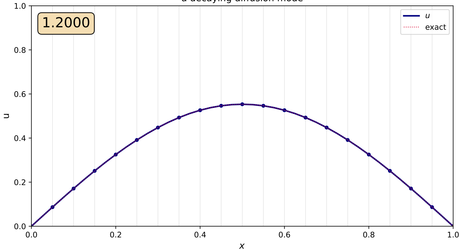
a decaying diffusion mode
