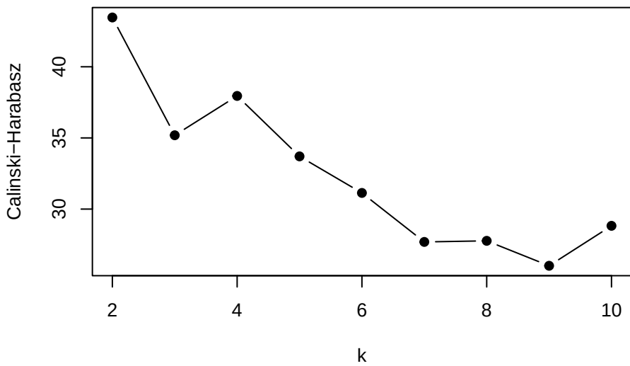
Calinski-Harabasz
