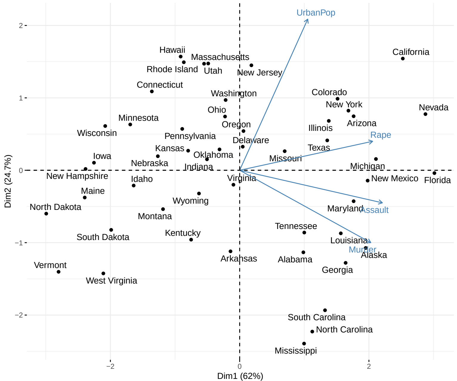
PCA – Biplot
