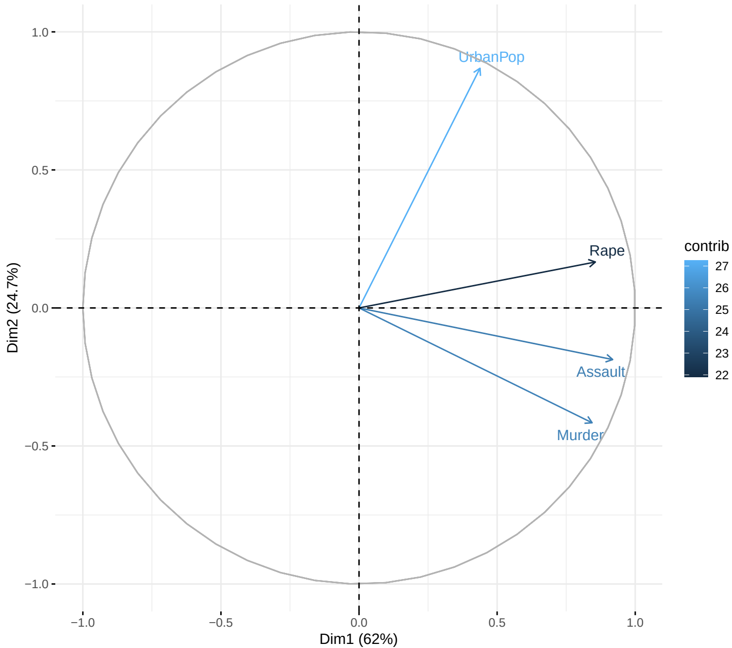
Variables – PCA
