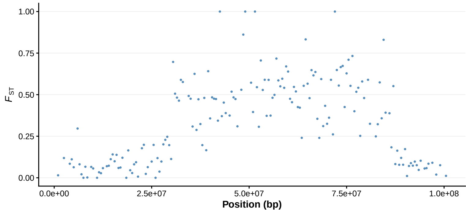
fst CRT AA vs CRT RR Omy05
