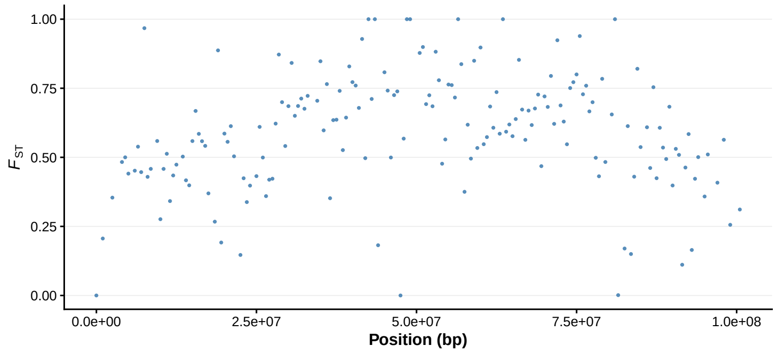
fst CRT AA vs WCT Omy05
