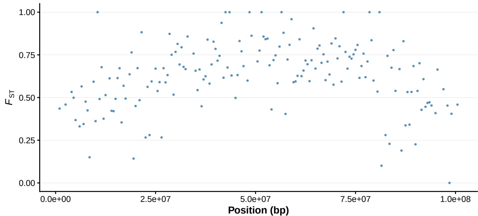
fst CRT AA vs YCT Omy05
