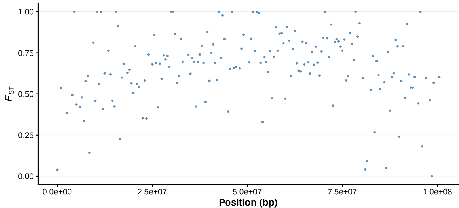
fst IRT vs YCT Omy05
