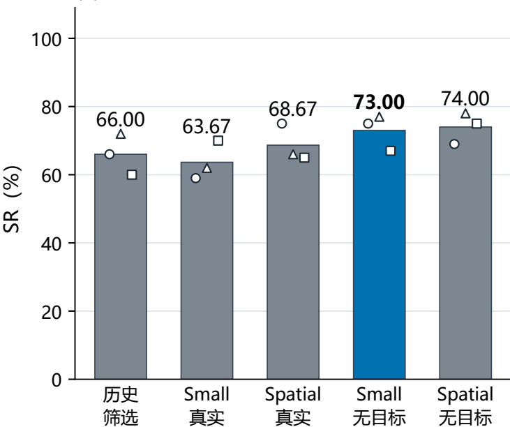
(a) 固定 val100×3: 当前默认来源
