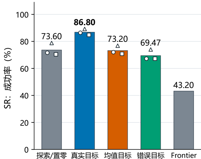
(a) 固定test250×3
