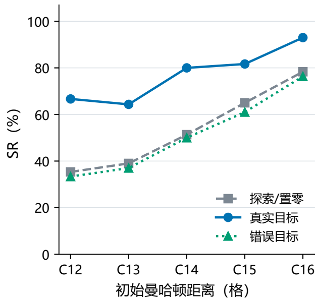
(a) 每档100题×3
