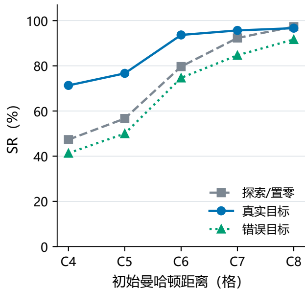
(a) 每档100题×3
