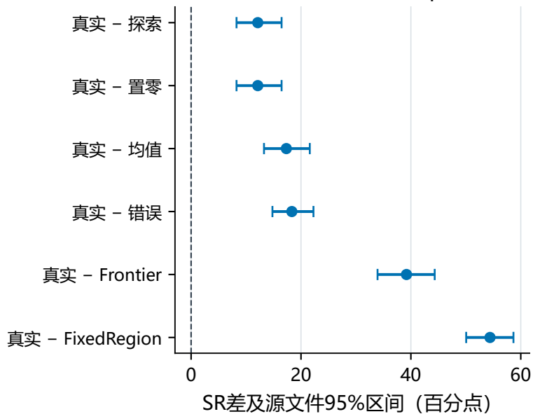
(b) 20源文件成组bootstrap
