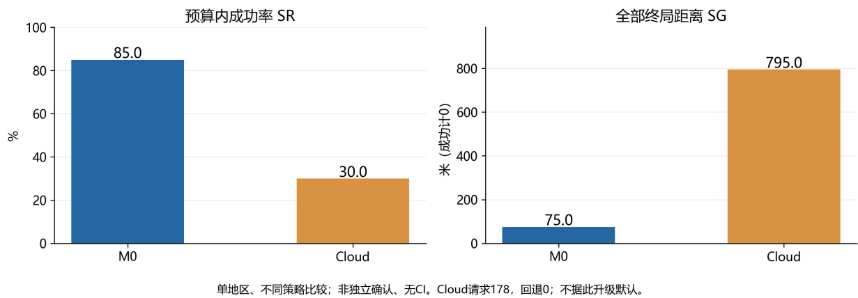
已消费开发区20题同题对照 5×5 / B10 / seed0
