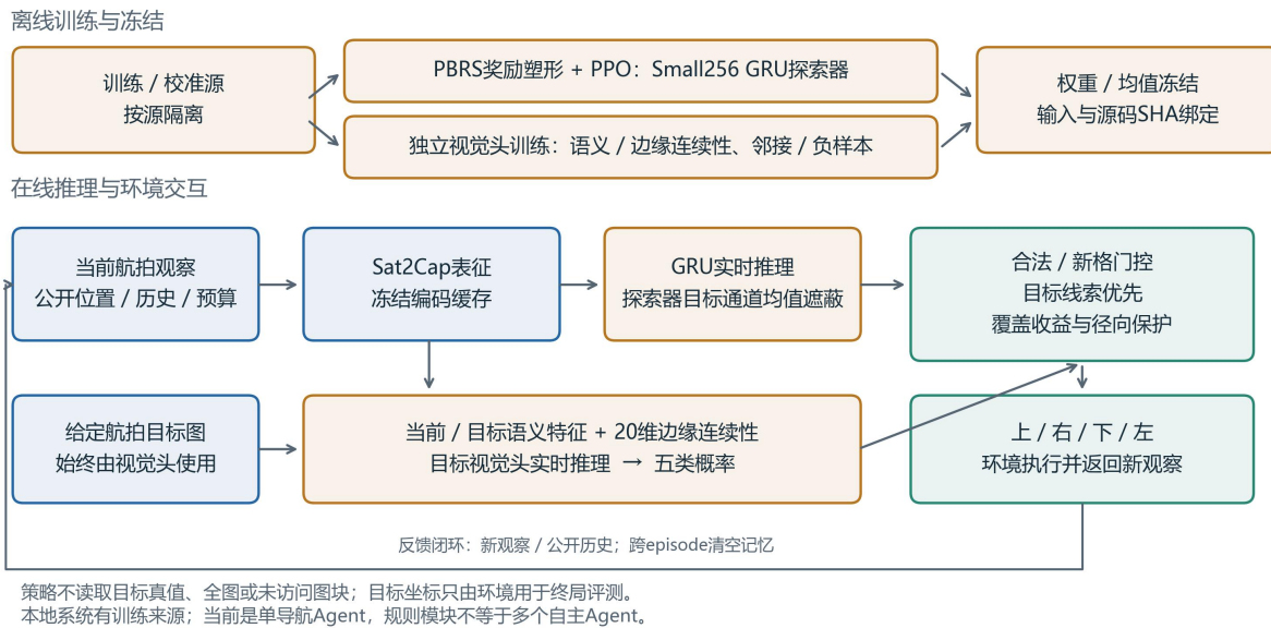
图 1 训练与在线推理分开。平台复用封存图像编码缓存，而 GRU 和视觉头每一步真正 forward；历史回放模式不推理。目标真值只供环境终局评测，不进入策略。
