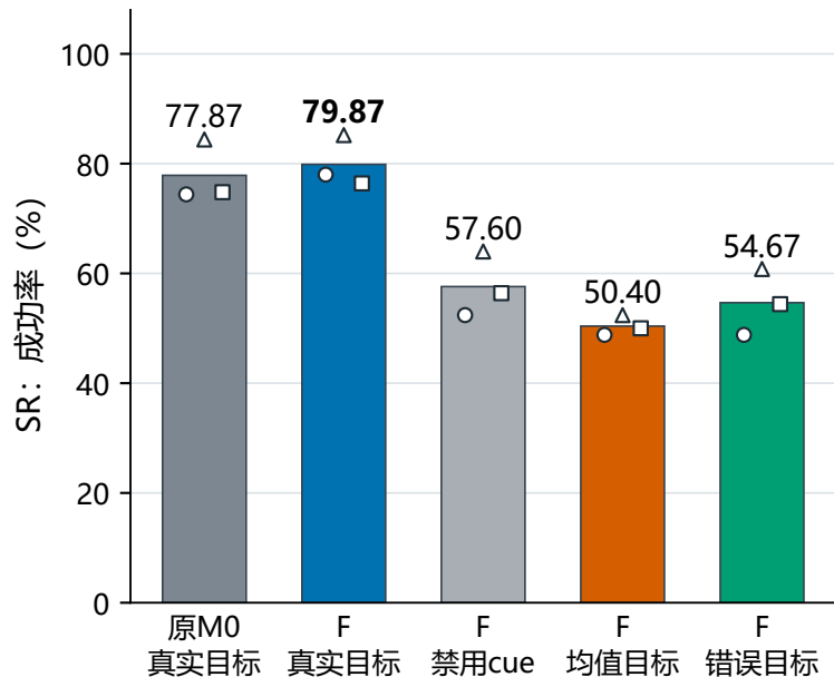
(a) 同题SR提升2.00个百分点
