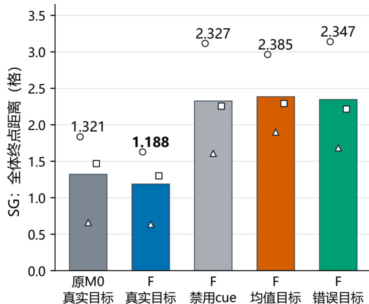
(b) 主对照与目标干预
