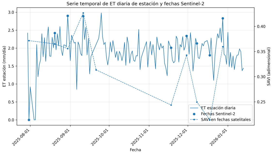
Figura 3: Disponibilidad temporal de datos de estación y fechas satelitales útiles para el análisis.
