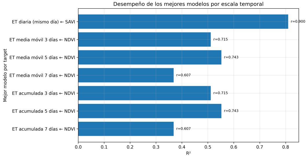
Figura 5: Comparación de modelos e índices espectrales evaluados.
