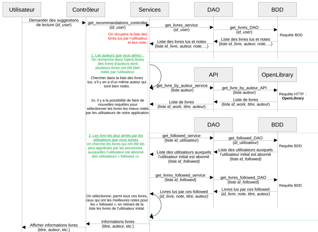
Figure 5: Diagramme de séquence : demander des recommandations
