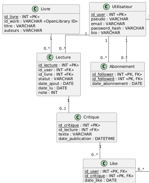
Figure 1: Modèle de données
