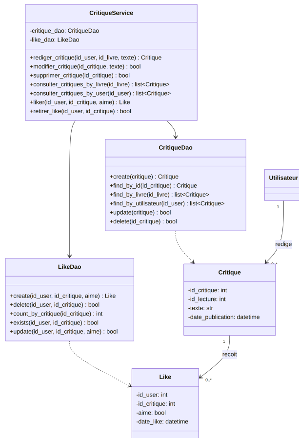
Figure 3: Diagramme de classes : critique
