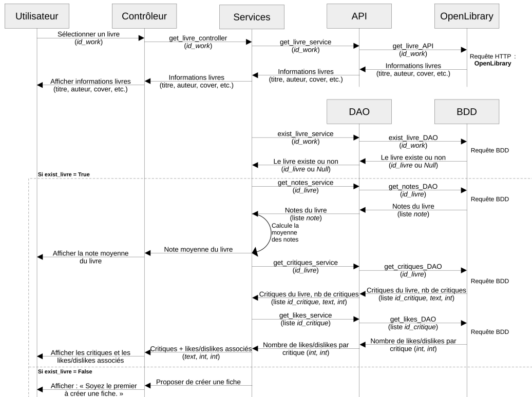
Figure 4: Diagramme de séquence : sélectionner un livre
