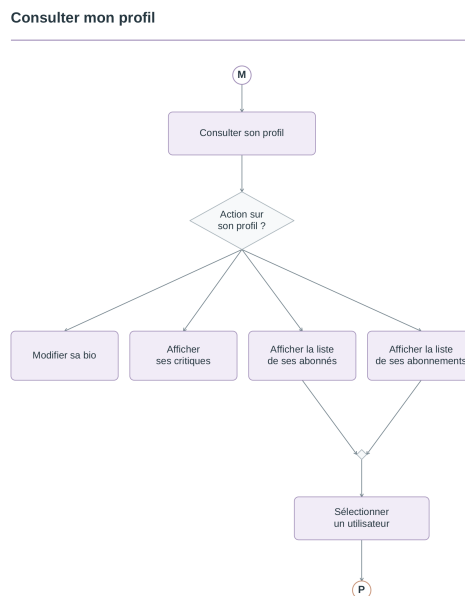
Figure 4: Diagramme d'activité : gestion du profil personnel
