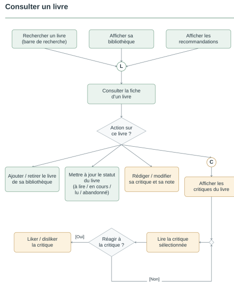
Figure 5: Diagramme d'activité : consultation d'un livre
