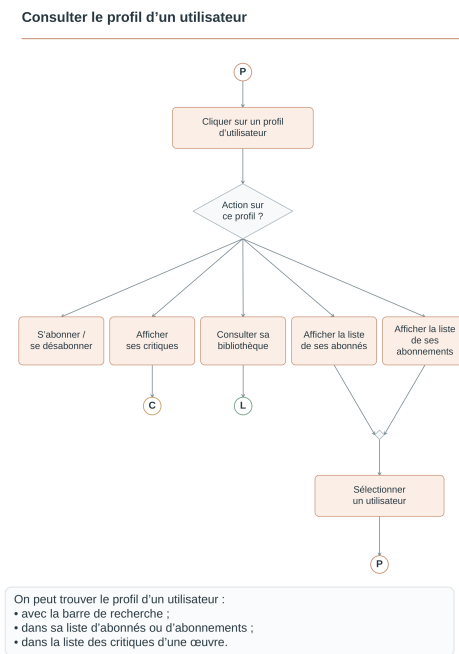
Figure 6: Diagramme d'activité : consultation du profil d'un utilisateur
