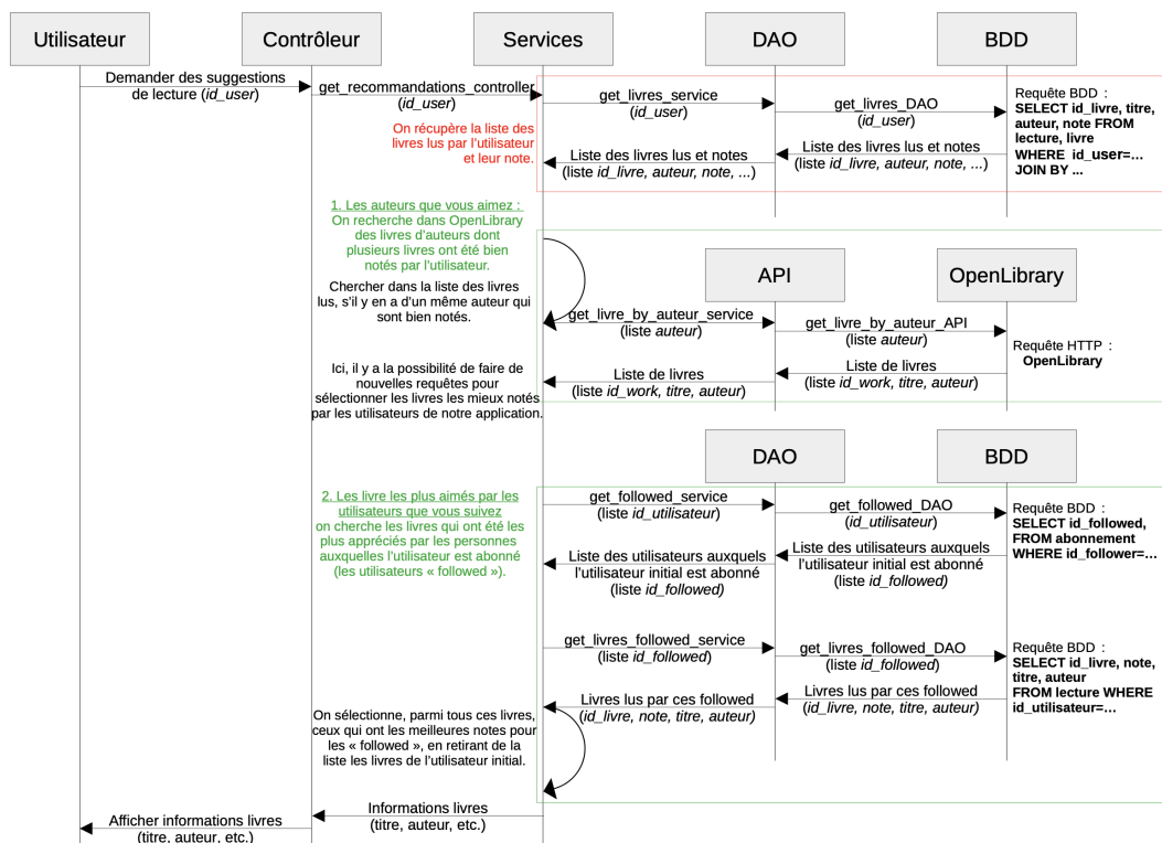
Figure 13: Diagramme de séquence : demander des recommandations
