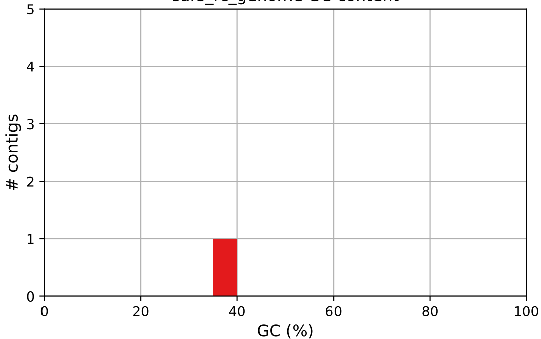
sars_rc_genome GC content
