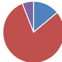
Leerjaar 4
