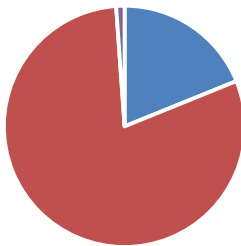
Leerjaar 3
