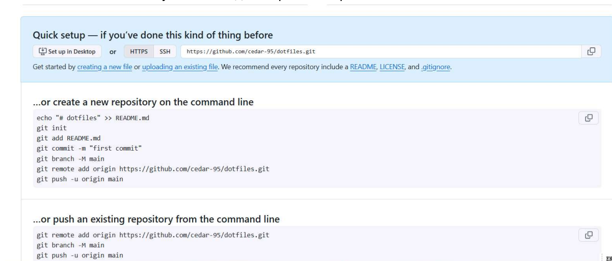
Рисунок 2: Создание репозитория dotfiles на GitHub
