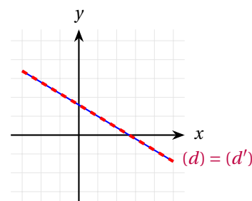
Droites confondues Infinité de solutions
