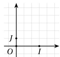
Repère orthogonal
