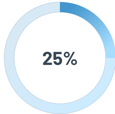
Setosa
