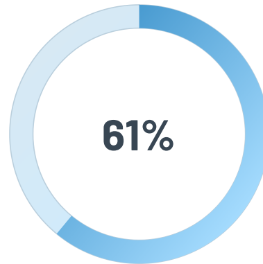
Versicolor
