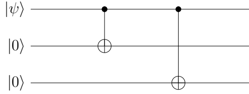
FIGURE 9 – Encodage du qubit logique dans le code correcteur à trois qubits.
