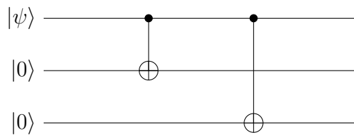
FIGURE 12 – Encodage du qubit logique dans le code correcteur à trois qubits.
