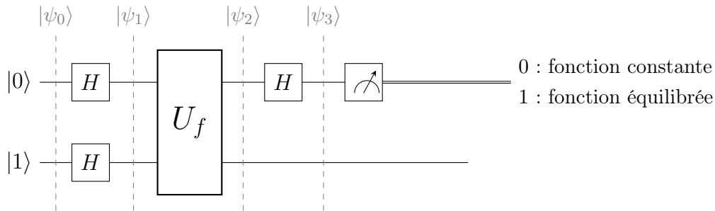
FIGURE 11 – Circuit quantique de l'algorithme de Deutsch.
