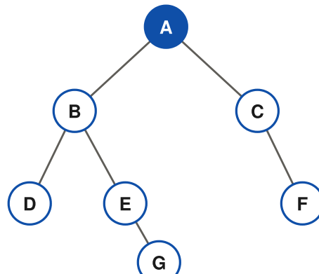
Un arbre de taille 7 et de hauteur 4.
