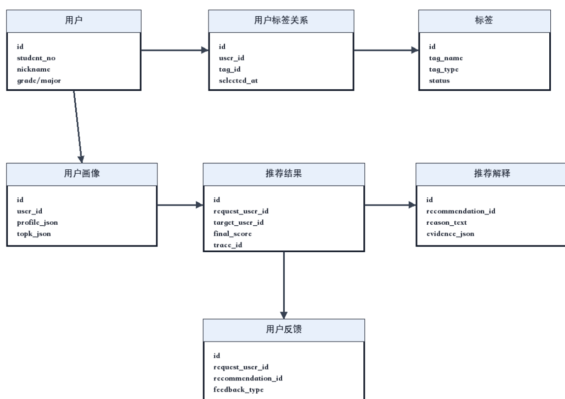
图 4-5 数据存储逻辑模型示意图
