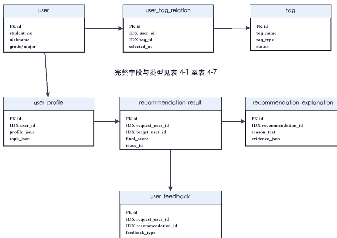
数据存储物理模型示意图
