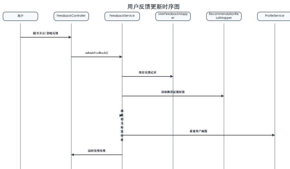
图 5-11 用户反馈更新时序图
