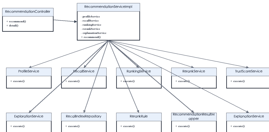
匹配推荐生成模块类图
