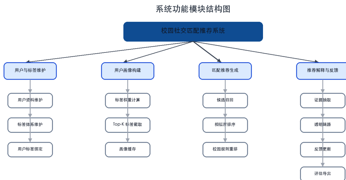
图 4-2 系统功能模块结构图
