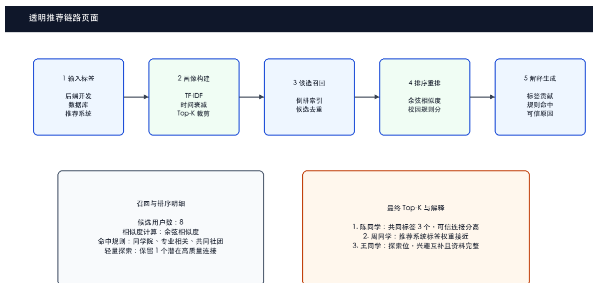
图 5-8 透明链路页面推荐生成阶段界面
