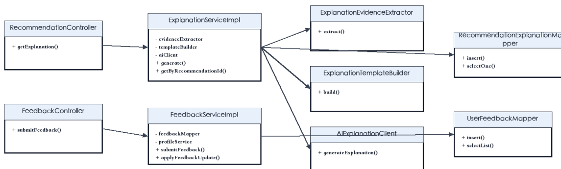
推荐解释与用户反馈模块类图
