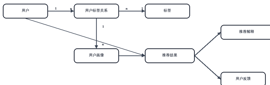
图 4-4 数据存储概念模型示意图
