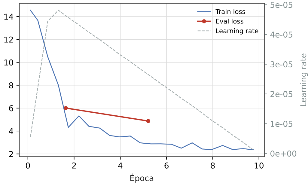
Loss de treino e validação
