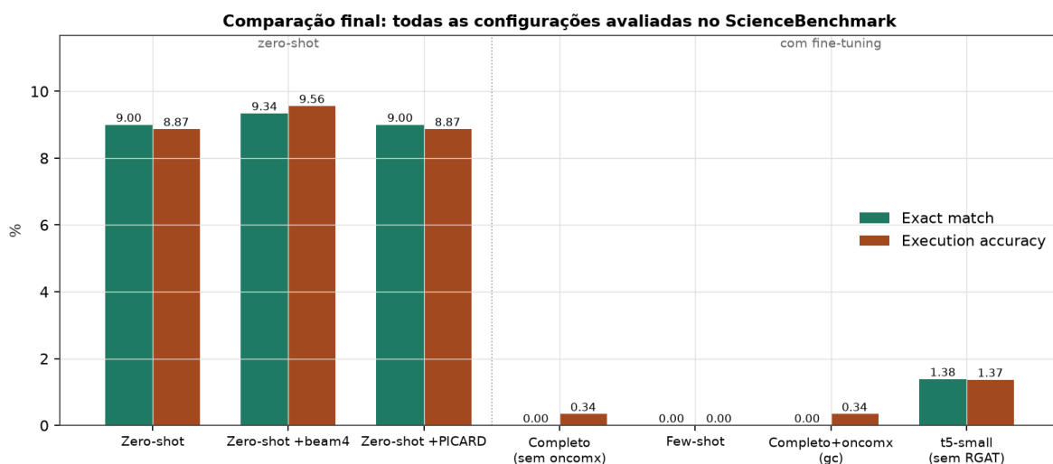
Figure 1: Exact match e execution accuracy de todas as sete configurações.
