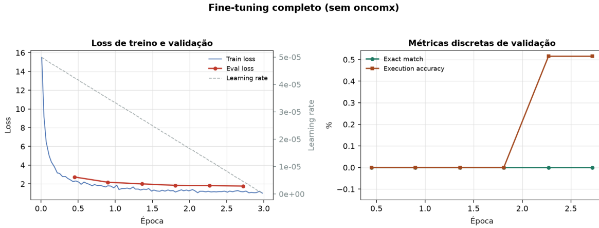
Figure 3: Fine-tuning completo (sem oncomx) – curvas de treino.
