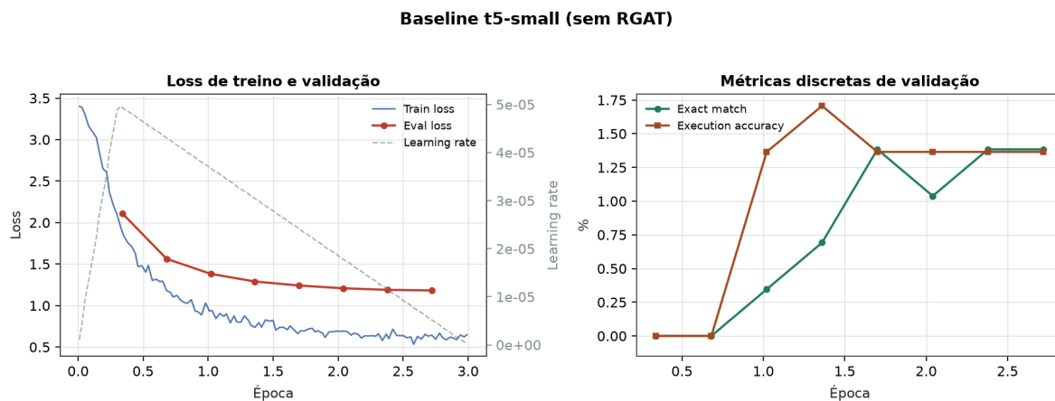
Figure 9: Baseline t5-small sem RGAT – curvas de treino.
