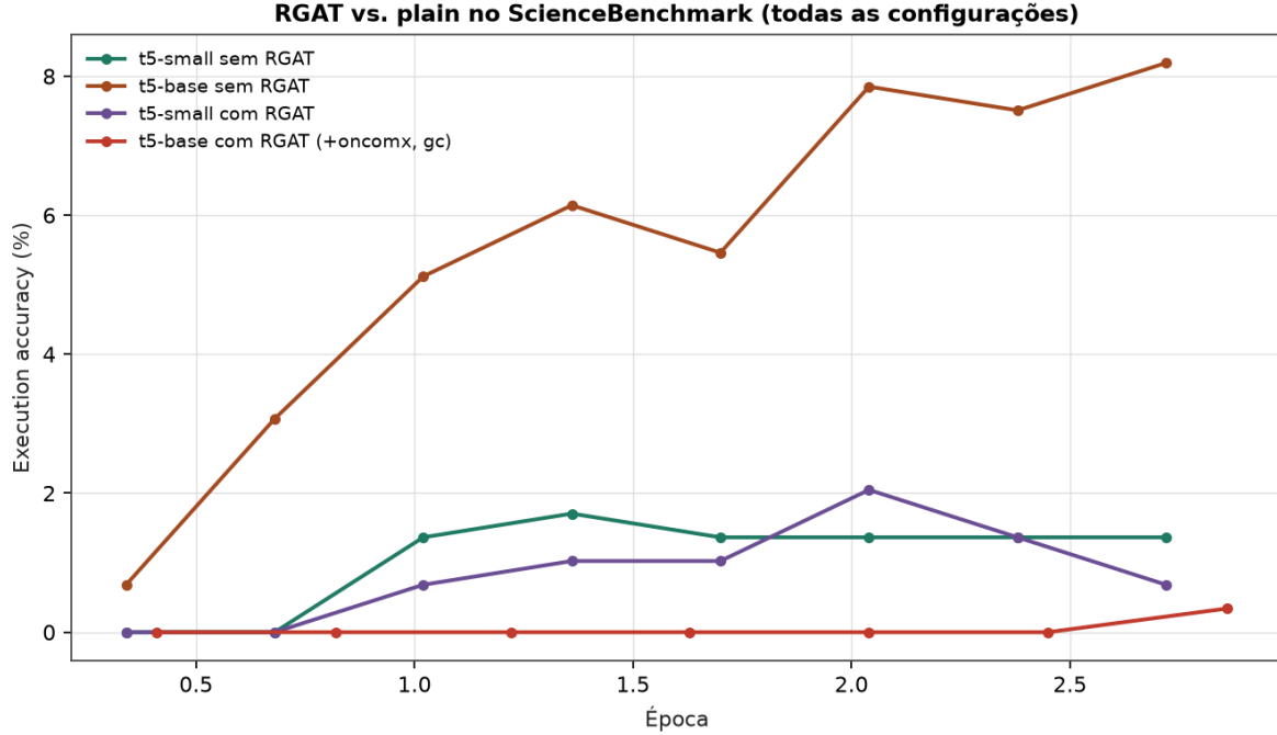
Figure 12: Execution accuracy de validação, as quatro configurações do ScienceBenchmark (t5-small/t5-base \times com/sem RGAT). Detalhes completos em estudo/scibench_ablation.tex .
