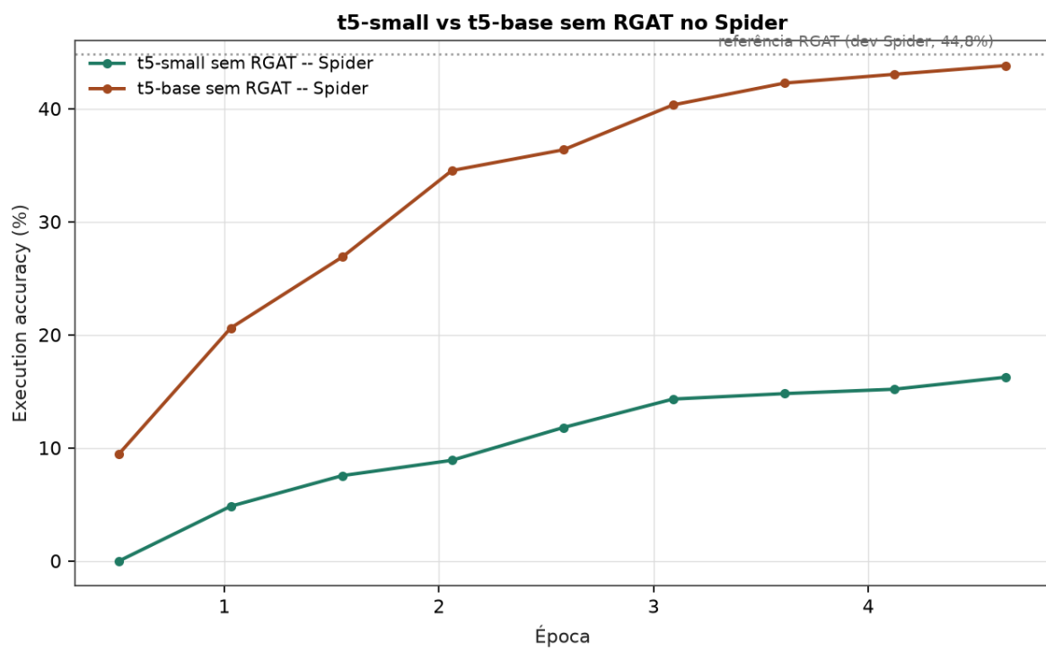
Figure 13: Execution accuracy de validação no Spider, t5-small vs. t5-base sem RGAT, com a referência RGAT marcada. Detalhes completos em estudo/spider_ablation.tex .
