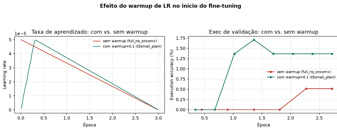
Figure 3: Efeito do warmup de LR: taxa de aprendizado (esquerda) e execution accuracy de validação (direita), comparando a única configuração sem warmup ( full_no_oncomx ) contra uma configuração com warmup=0,1 ( t5small_plain ).
