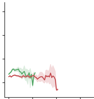
Llama-3.2-1B-Instruct
