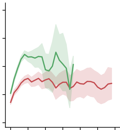
Llama-3.2-3B-Instruct
