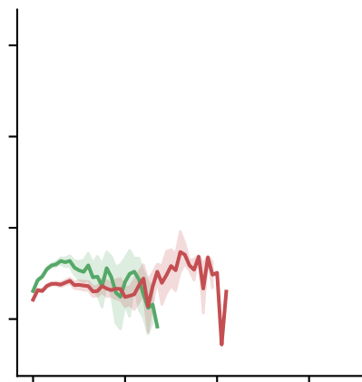
Llama-3.2-3B-Instruct
