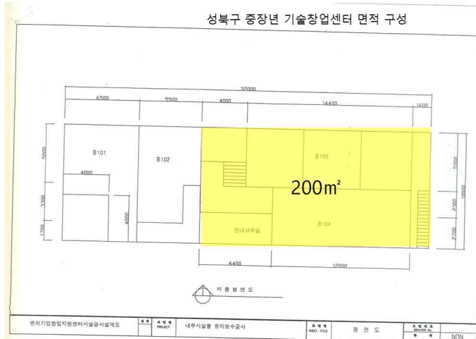
센터 평면도
