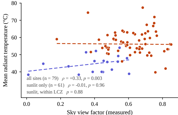
(d) Sky view factor vs T_{mrt}
