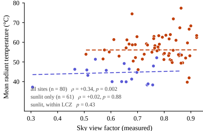
(d) Sky view factor vs T_{mrt}
