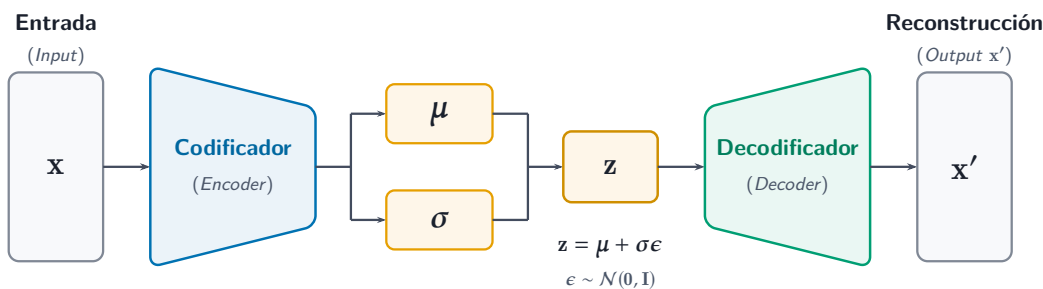
Figura 2.6: Diagrama esquemático del funcionamiento de un Autoencoder Variacional (VAE). Adaptado de [34].
