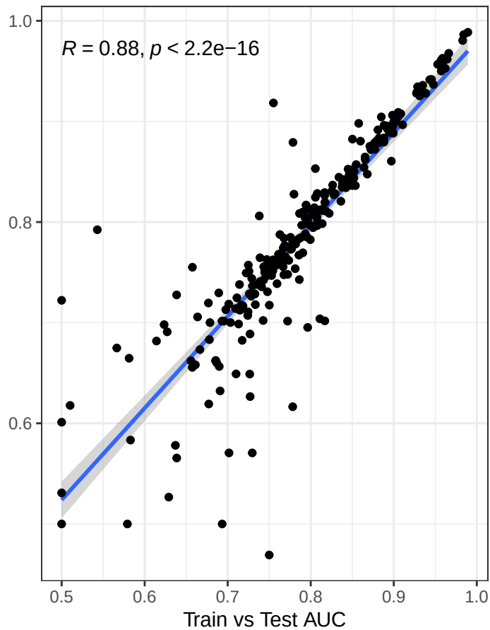
TRAIN AUC vs TEST AUC
