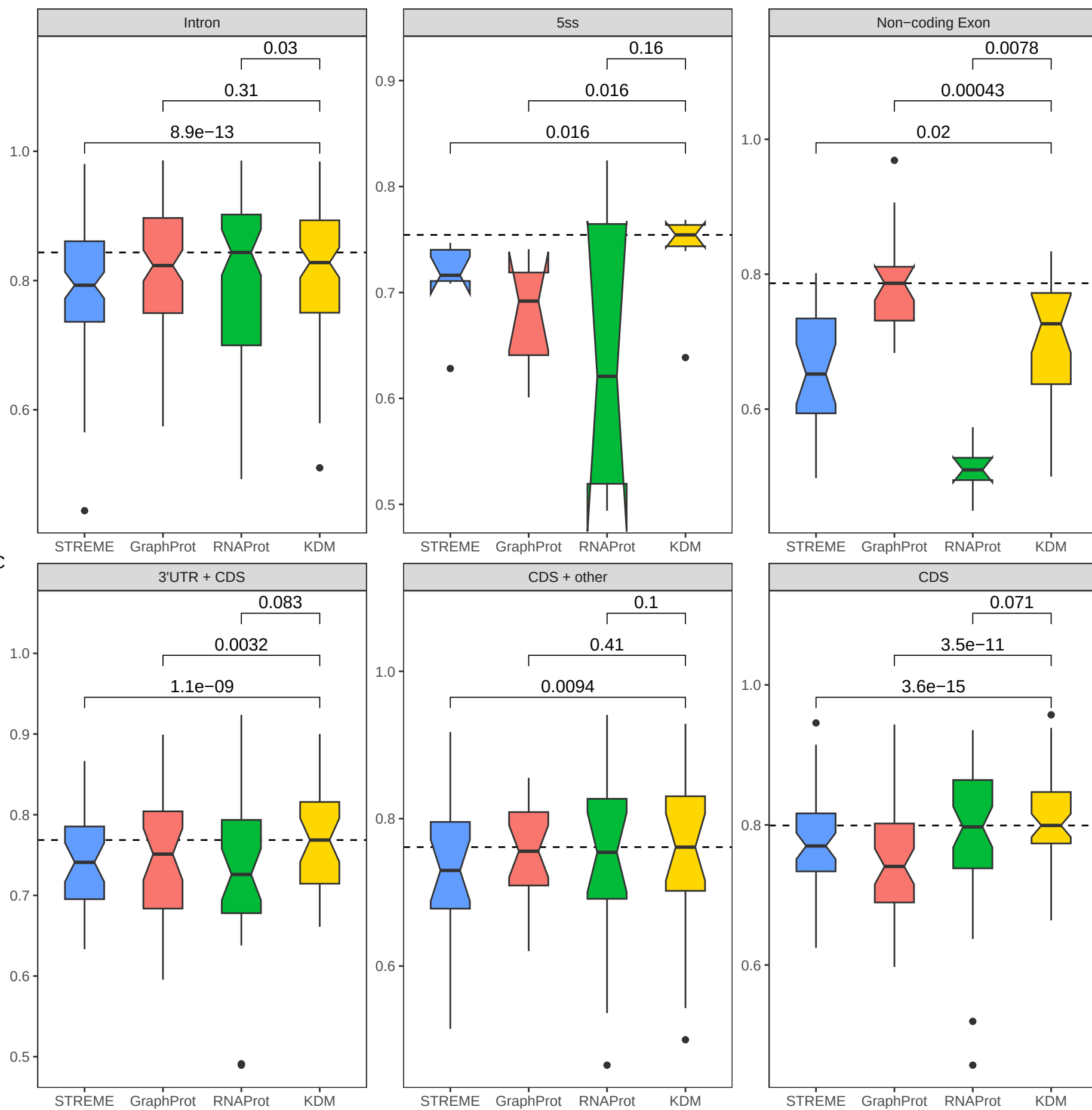
AUC distributions ~ VN_Classes
