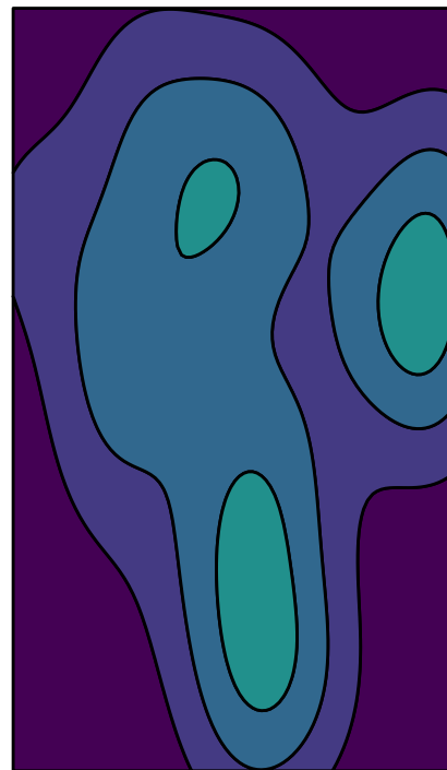
UTR3
