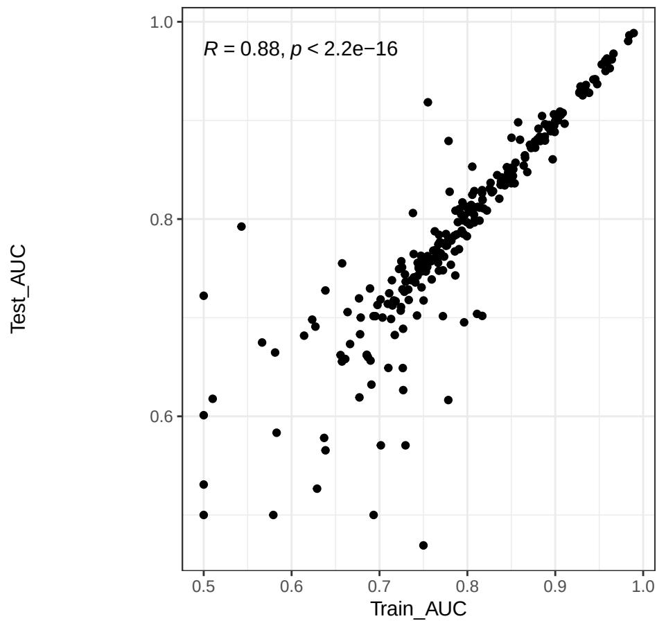
TRAIN AUC vs TEST AUC
