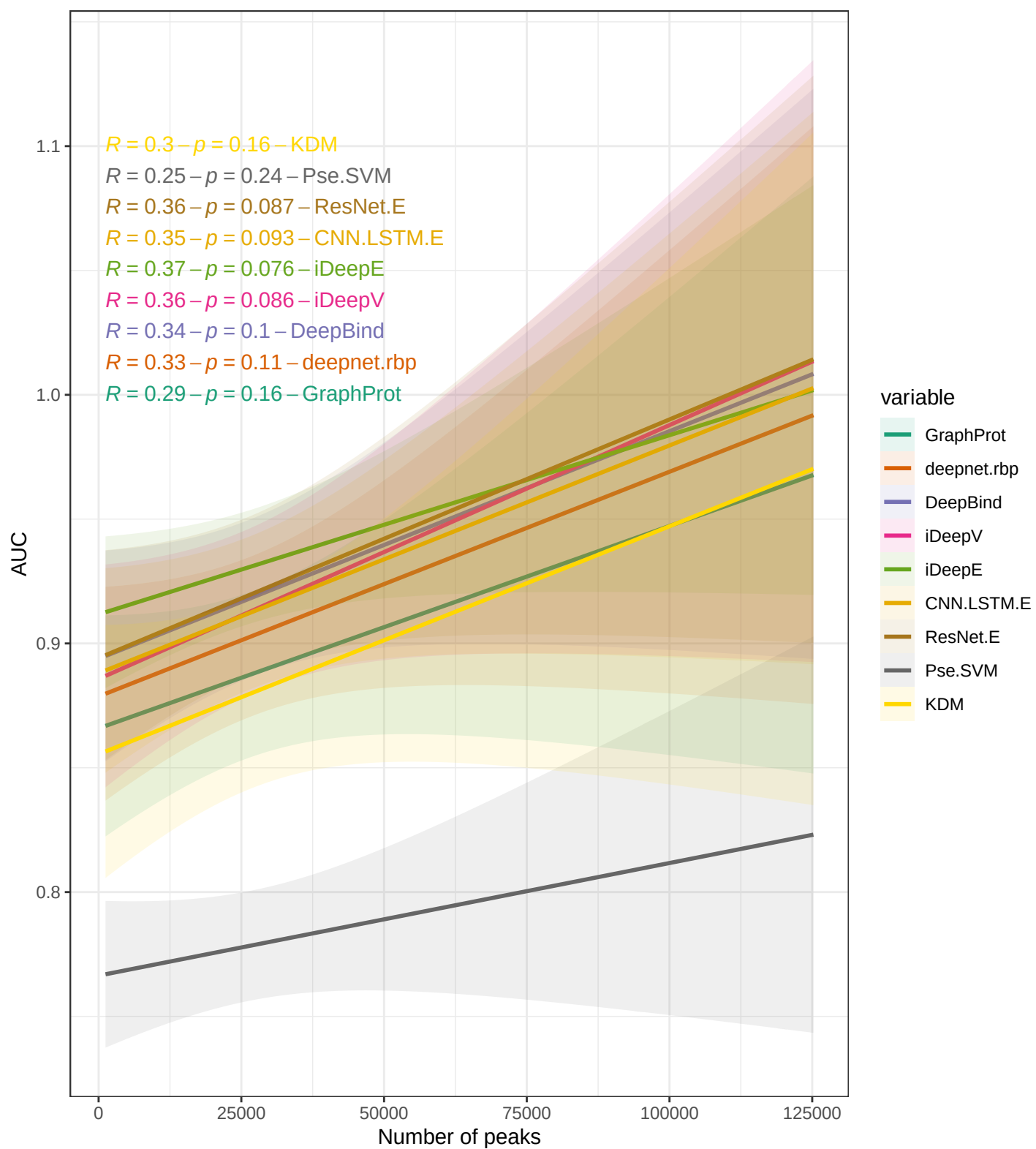
AUC ~ N.Peaks
