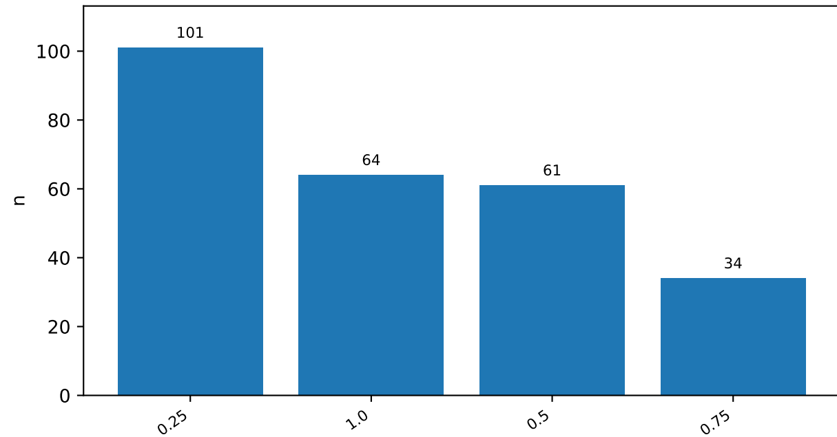
IHC
