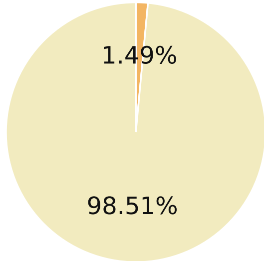
LLaMA-3.3-70B-Instruct-int4-gptq
