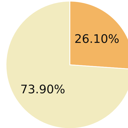
Qwen3-0.6B-int4-gptq
