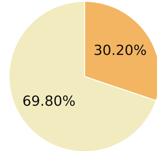
Gemma-3-1b-it-int4-gptq
