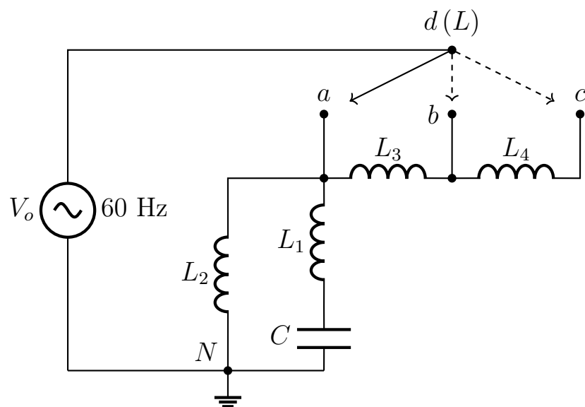
Figura 1: Esquema eléctrico de un ventilador de 3 velocidades.
