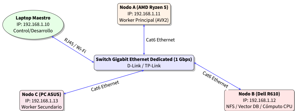
Figura 1: Plano de Red Lógico del Clúster de Procesamiento en Paralelo
